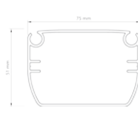
Vučni profil 75x51mm
