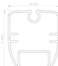
Horizontalni profil 45x51mm
